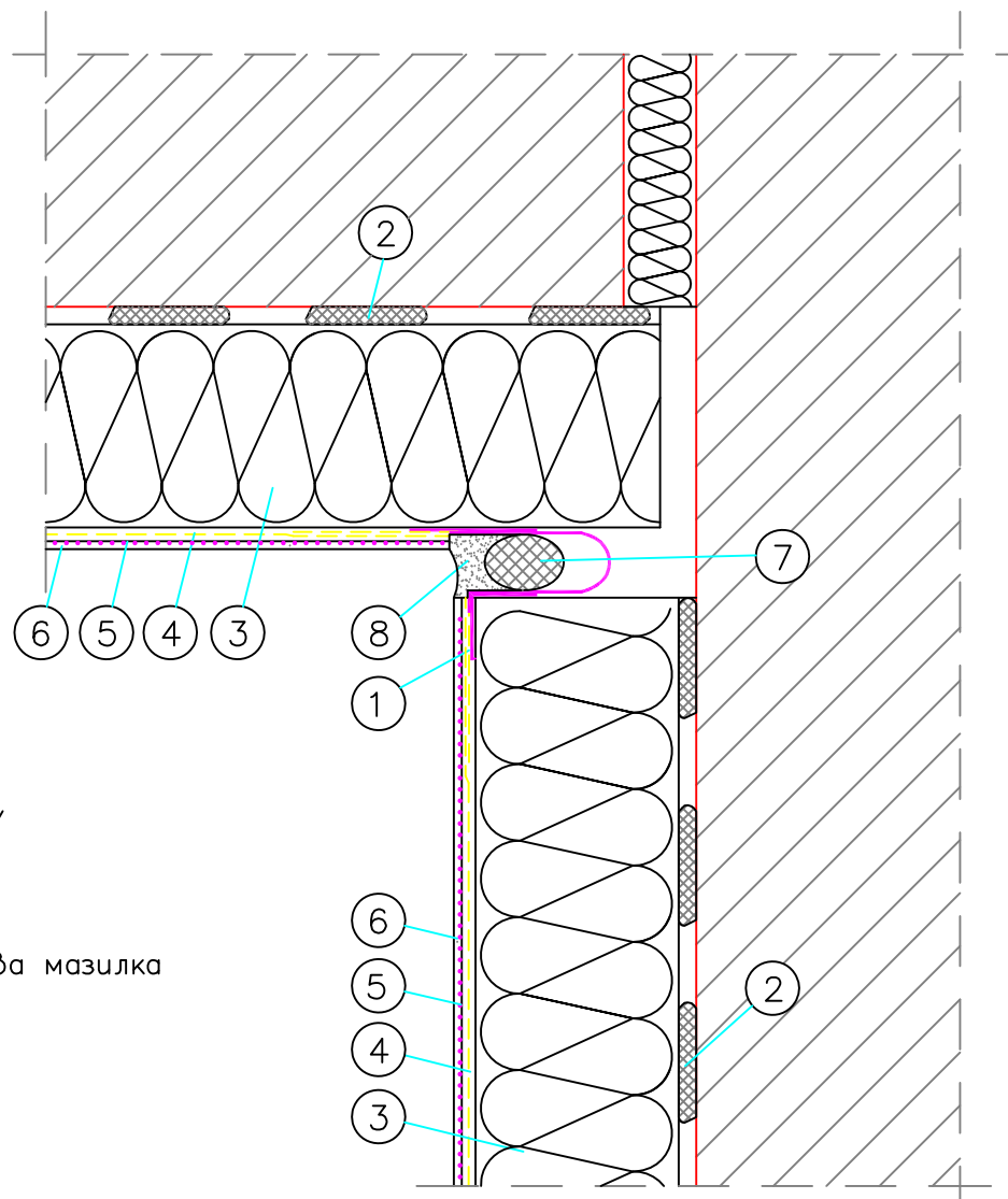
Fig. 7.25 Уплътняване на ъгъл на деформационна фуга с дилатационна лента – запълване с полиуретанов уплътнител
