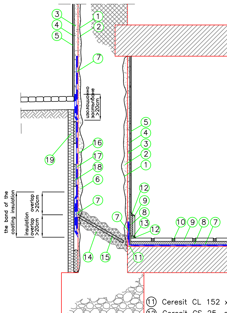
Fig. 6.3. Външен сондаж на стената срещу капилярна влага, измазване на стените и външна изолация
