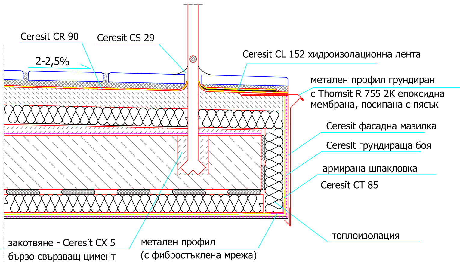
Фиг. 1.4с Външен край на балкона с топлоизолация
