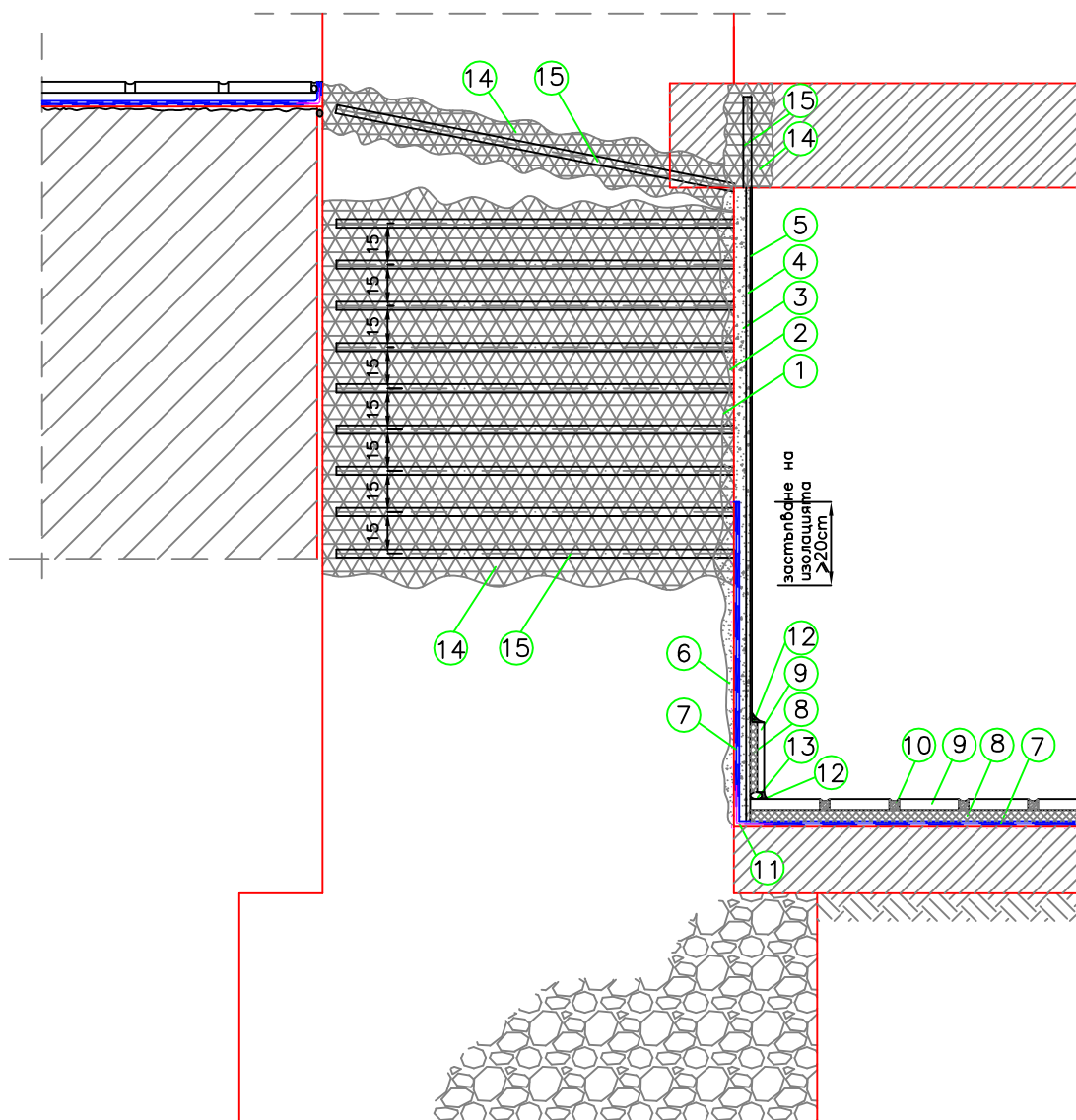
Fig. 6.6. Уплътняването на външната стена – инжекционен способ
