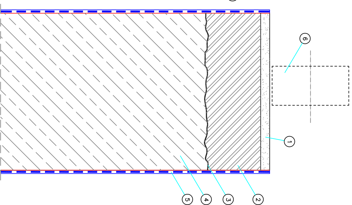
Fig. 5.8 Конструкцията на стената и пърното легло под колегелото на пречиствателя на вода в резервоара
