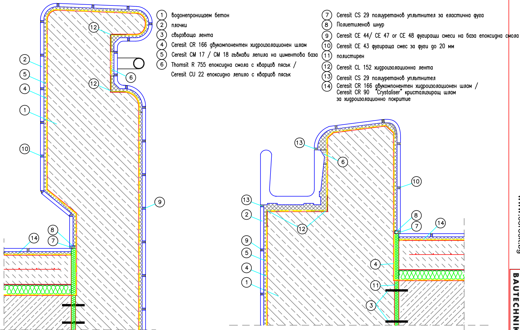
Fig. 4.5 Уплътняване на сифон тип "St. Moritz" в рехабилитационни басейн
