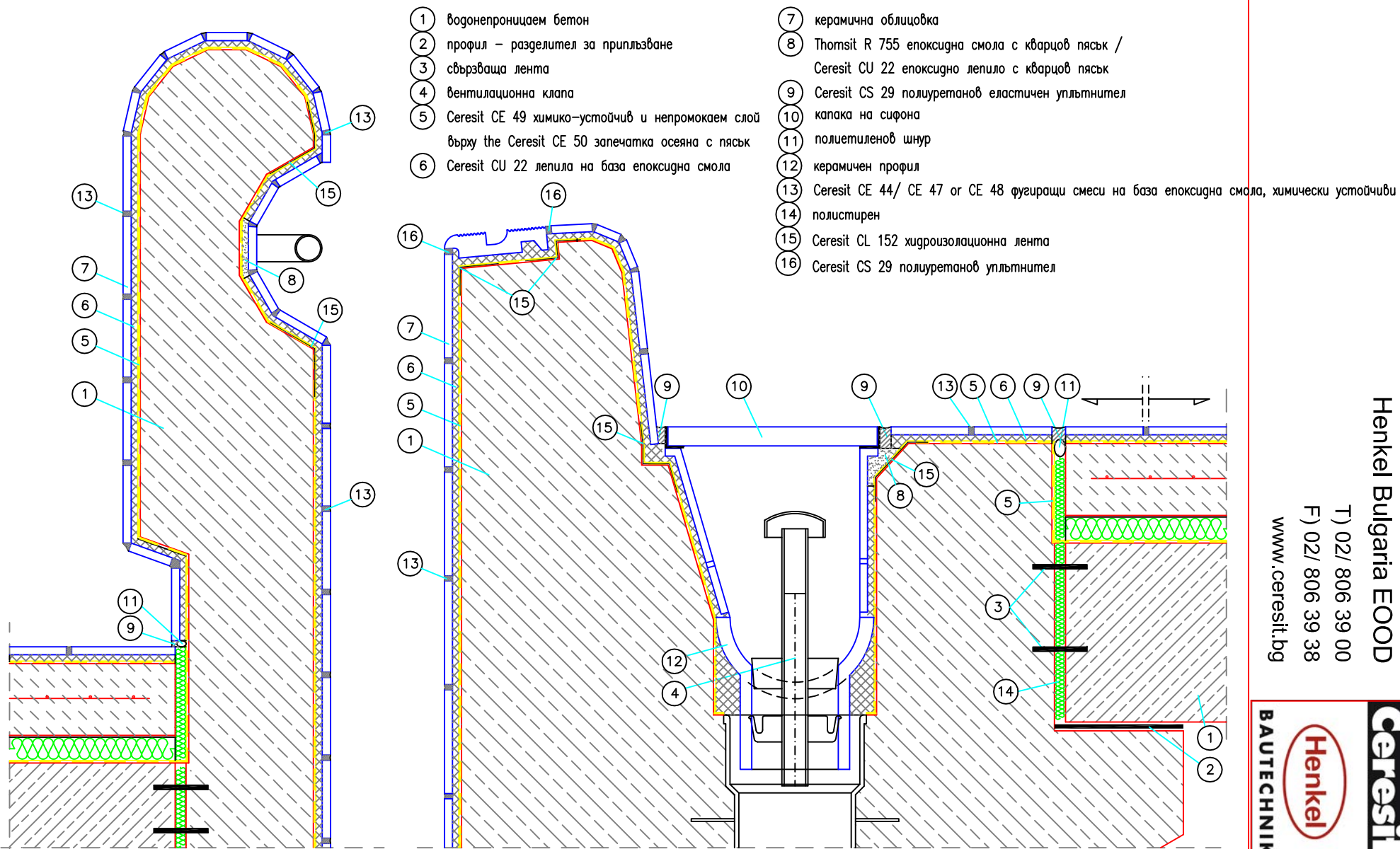
Fig. 4.6 Уплътняване на сифон тип "St. Moritz" в балнео басейн (водно pH <4,5 или pH >13,5)
