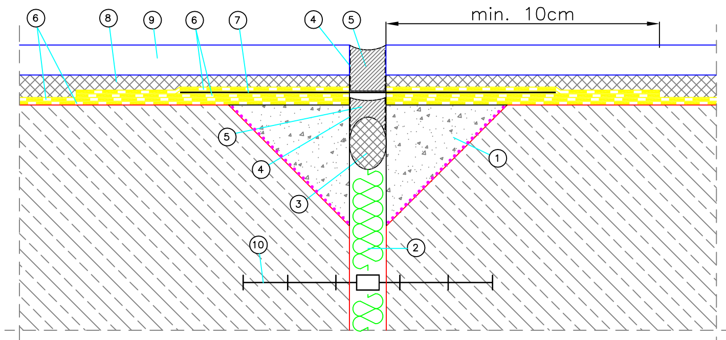
Fig. 4.8 Конструктивна разширителна fuga в плувен басейн
