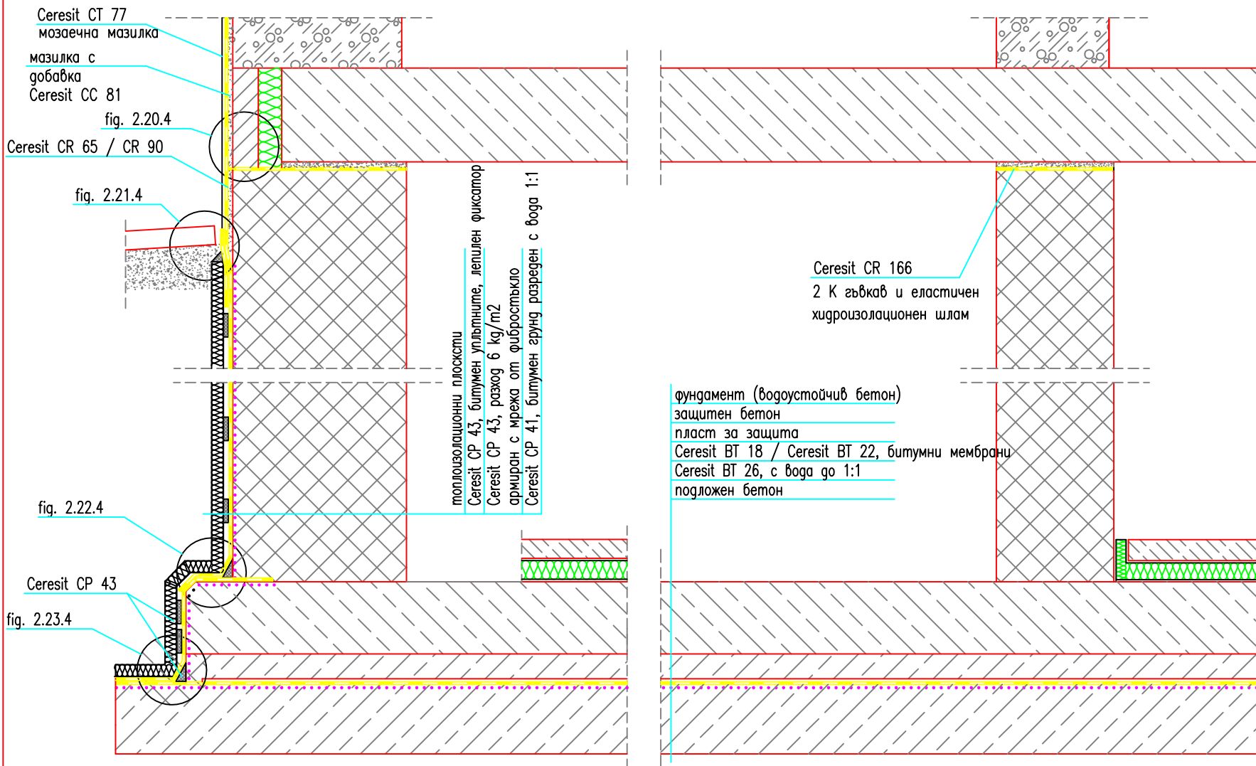
Fig. 2.4 Общ план
