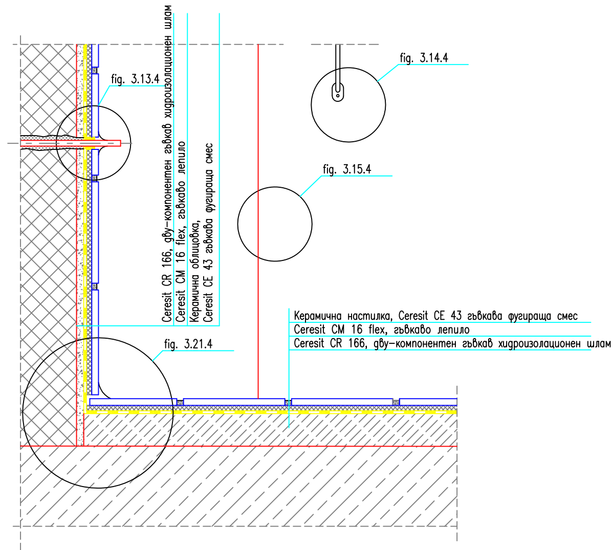
Fig. 3.4 Общ план
