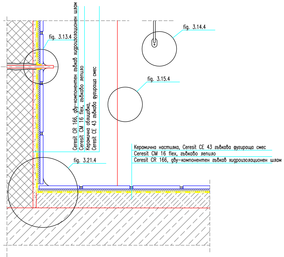
Fig. 3.4 Общ план
