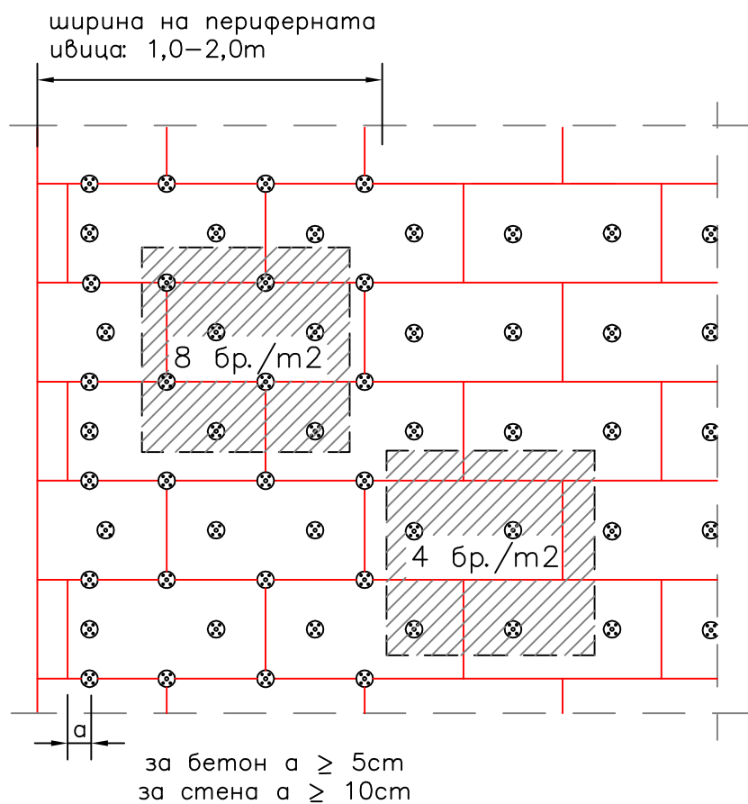
Fig. 7.1 Допълнително фиксиране на плочи от стиропор с елементи за механично закрепване около външните ъгли на сградите
