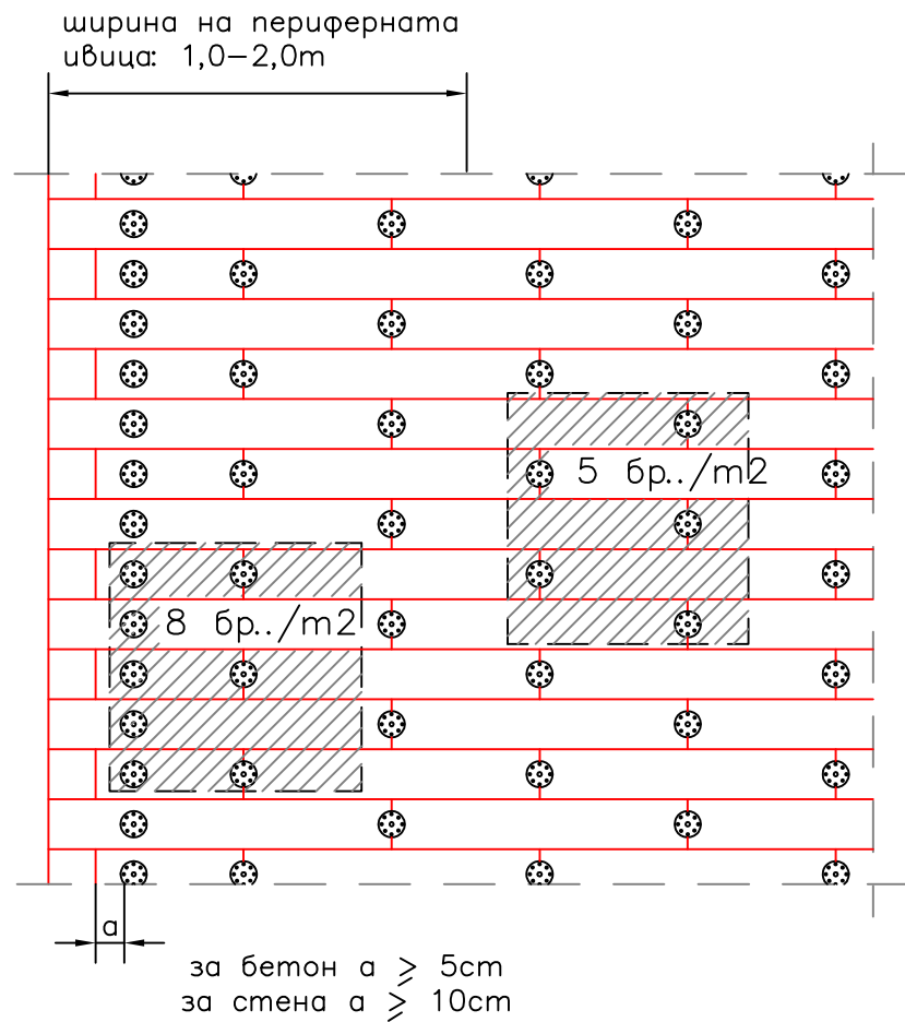
Fig. 7.3 Допълнително фиксиране на ламелни плочи с елементи за механично закрепване около външните ъгли на сградите
