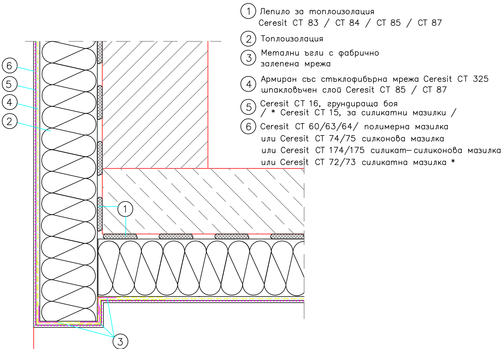
Fig. 7.9 Топлоизолационен на еркерен участък
