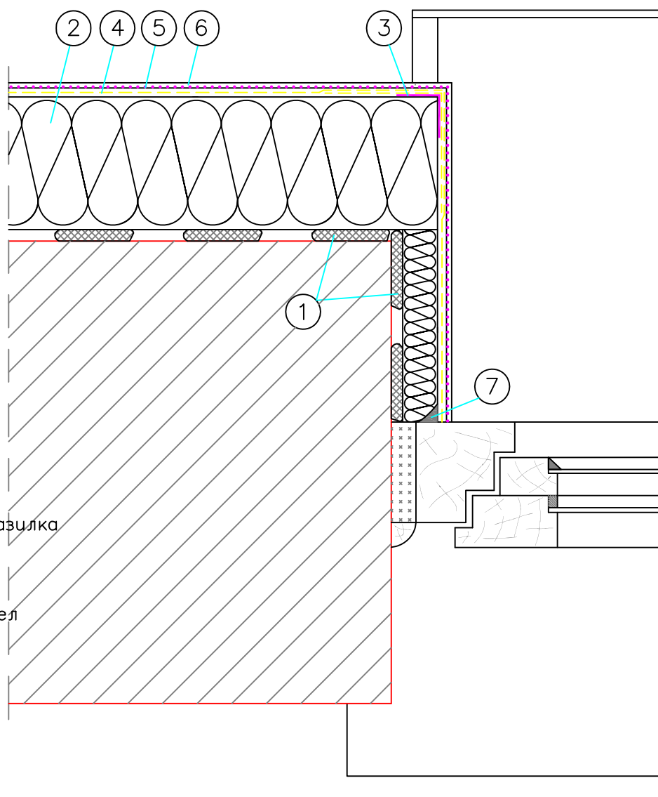
Fig. 7.13 Топлоизолиране на прозоречни рамки
