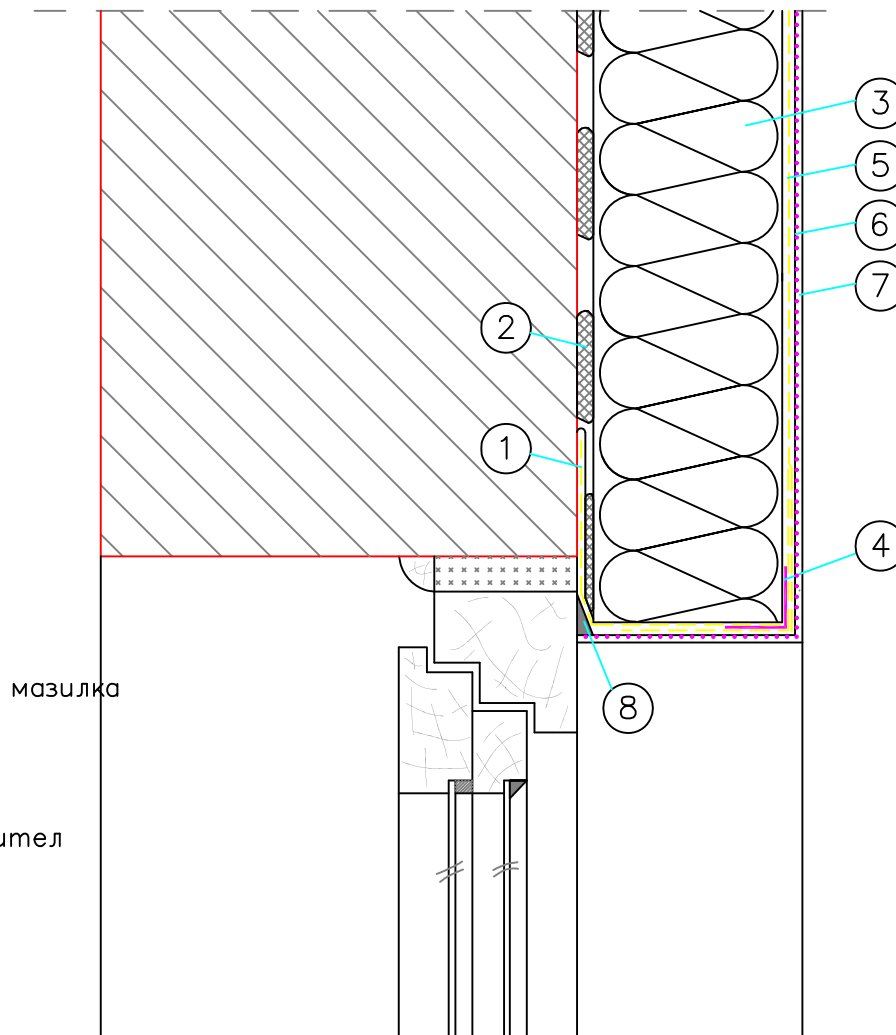
Fig. 7.16 Топлоизолиране на горе край на прозорец, разположен наравно с фасадата
