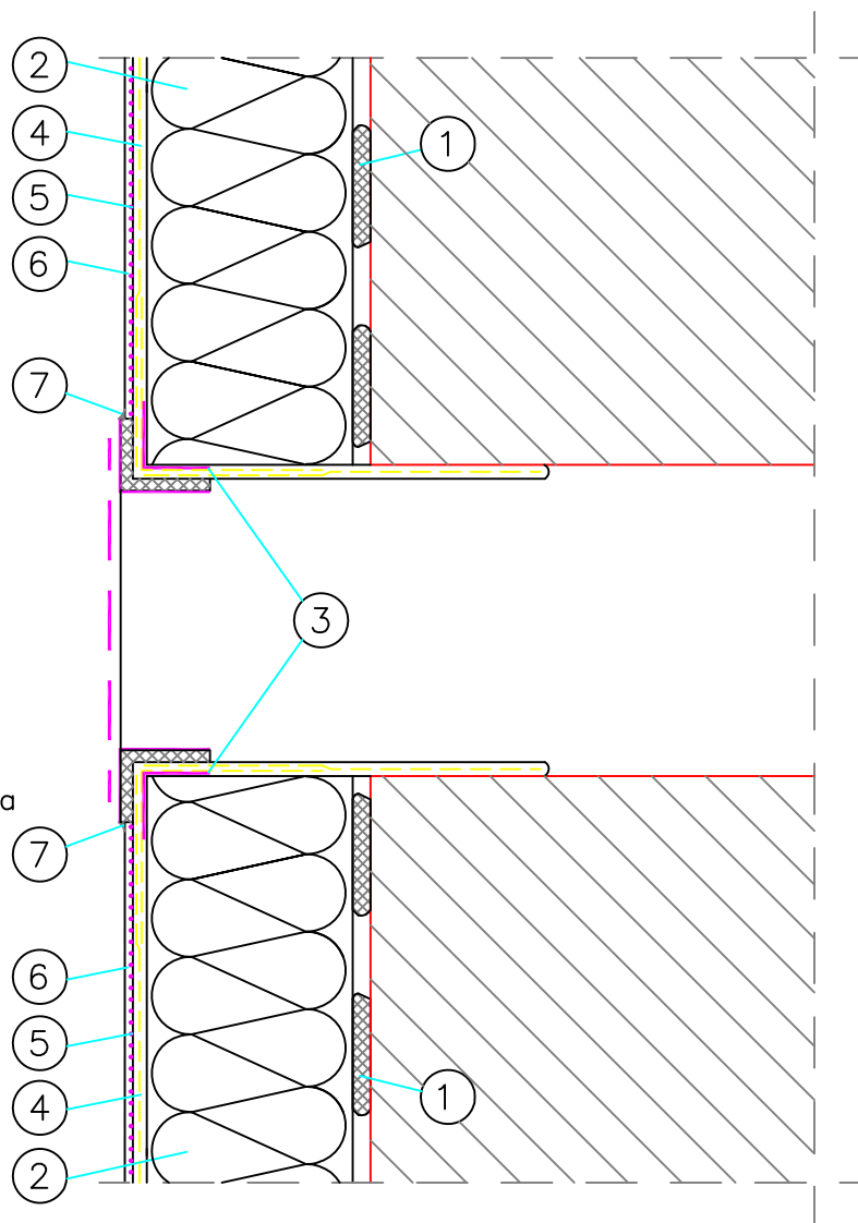
Fig. 7.22 Съединяване с въздуховод
