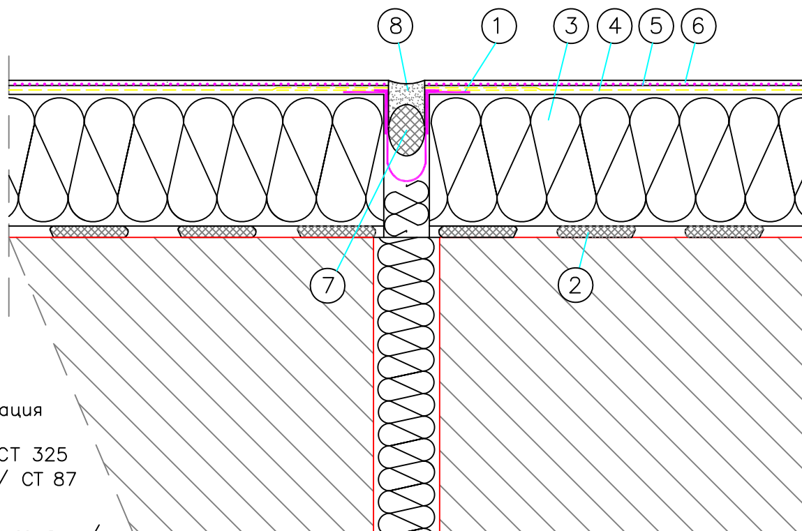
Fig. 7.23 Уплътняване на деформационна фуга с дилатационна лента – запълване с полиуретанов уплътнител
