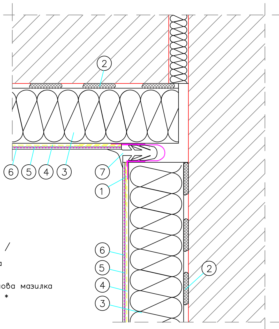
Fig. 7.26 Уплътняване на ъгъл на деформационна фуга с дилатационна лента – запълване с дилатационен профил
