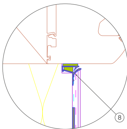
детайл мащаб 1:2
