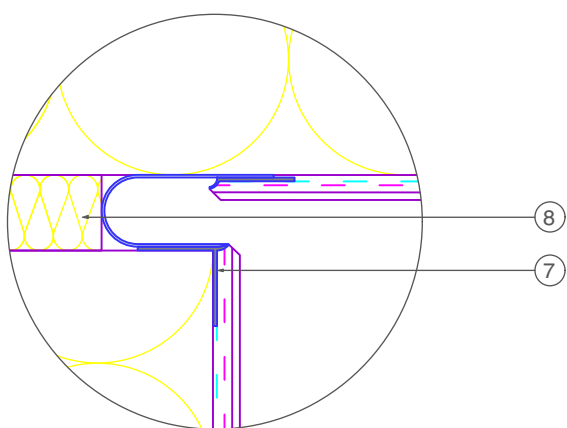
детайл мащаб 1:2
