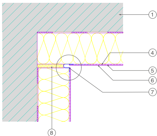
детайл мащаб 1:2
