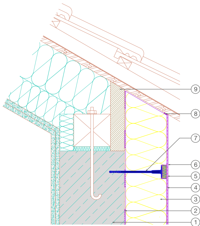
детайл мащаб 1:2
