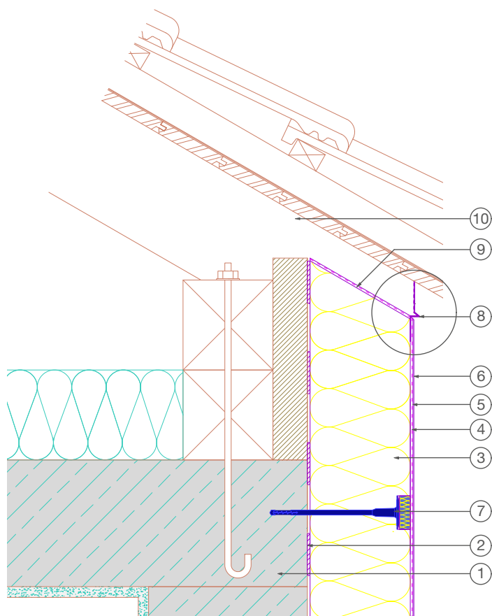
детайл мащаб 1:2
