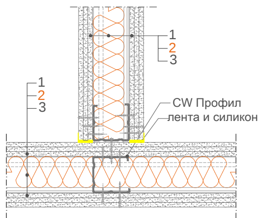
Т-връзка
