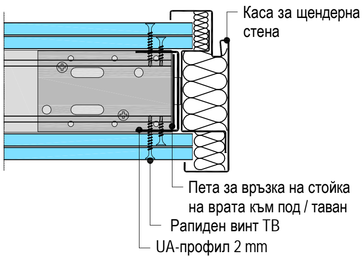
W362-E1-A Отвор на врата Вариант UA
