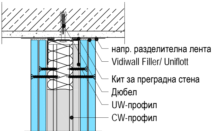
W362-VO1-A Връзка към таван
