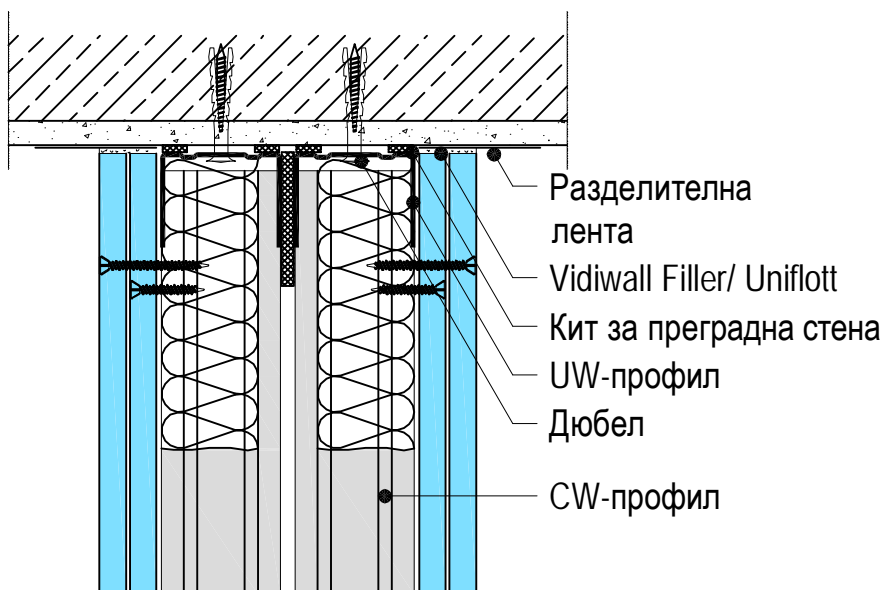
W365-VO1-A Връзка към таван
