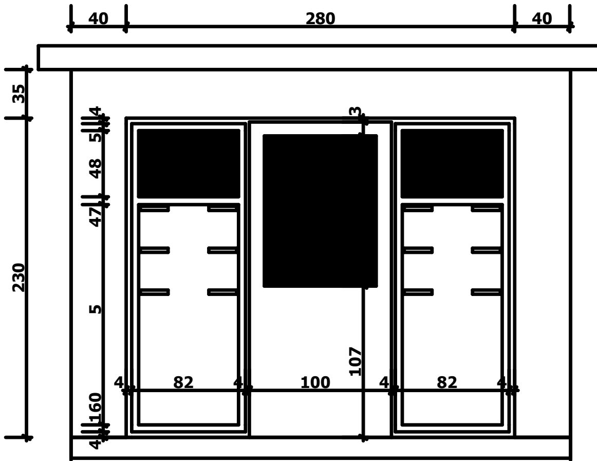
ИЗГЛЕД ОТВЪН
